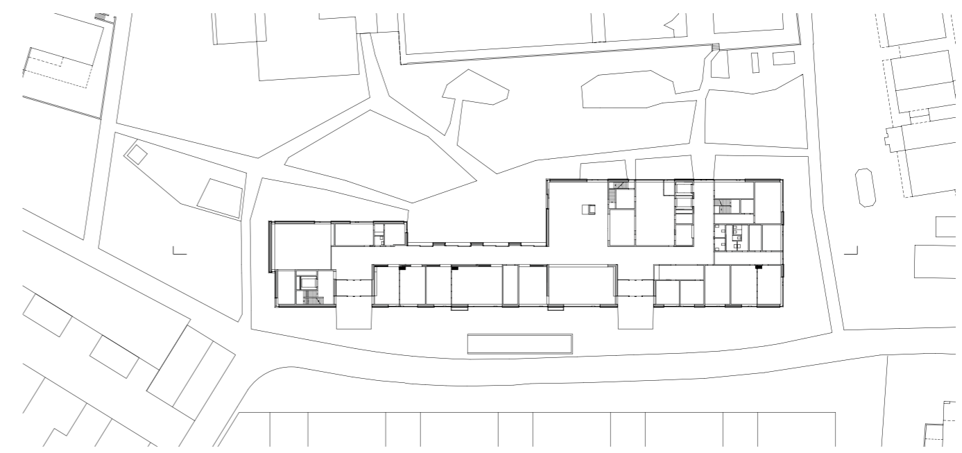
Erdgeschoss
